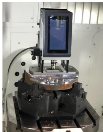
Mesure de rugosité d'une pièce par procédé optique
